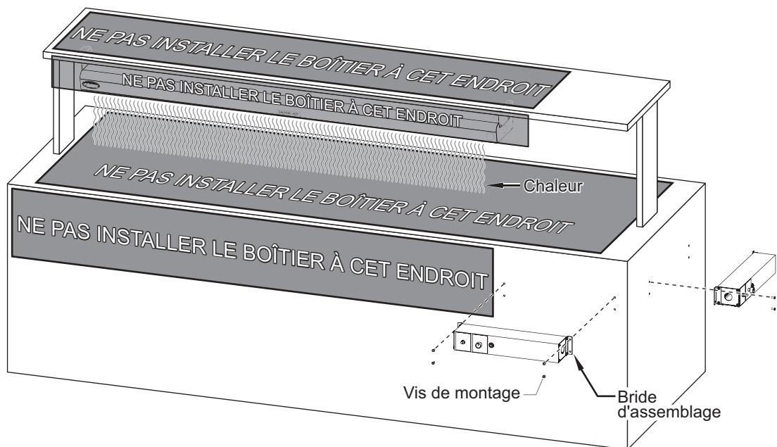
Emplacements pour l'installation du boîtier de commande à distance intégré
